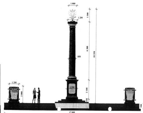
Проект стелы «Кронштадт – город воинской славы».
